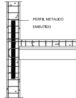
NUDO EXTREMO PILAR INTERRUPTO
