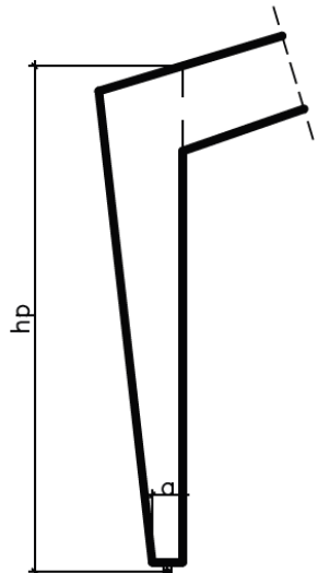
OPCIÓN DE APLOMADO INTERIOR
